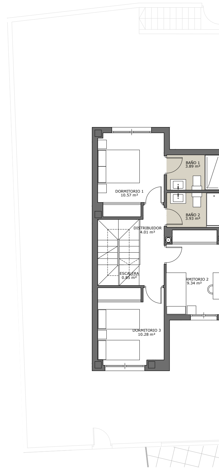
PLANTA PRIMERA
