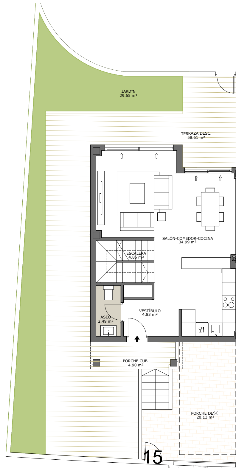
PLANTA BAJA
