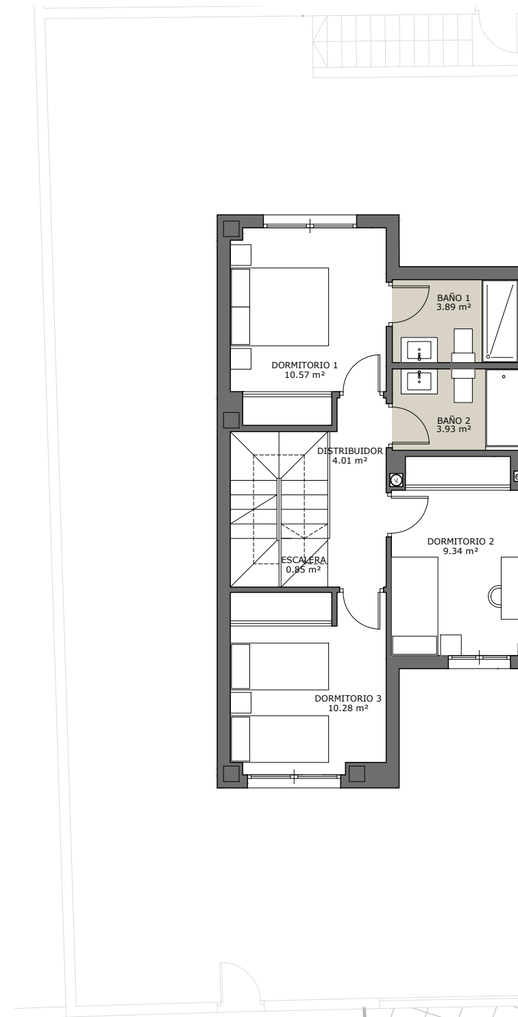
PLANTA PRIMERA
