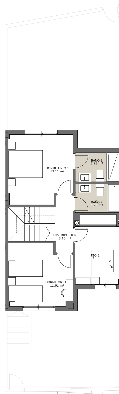
PLANTA PRIMERA
